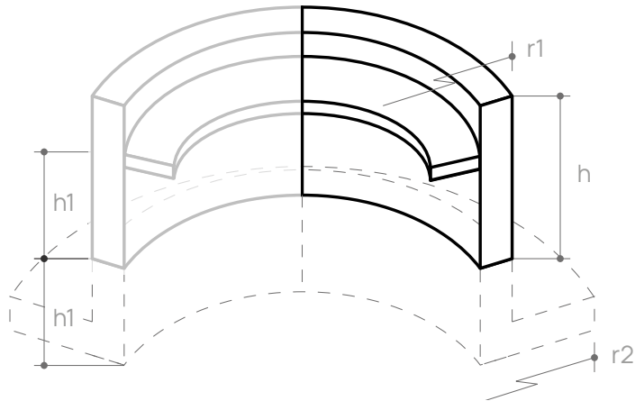
ПОДПОРНАЯ СТЕНКА
